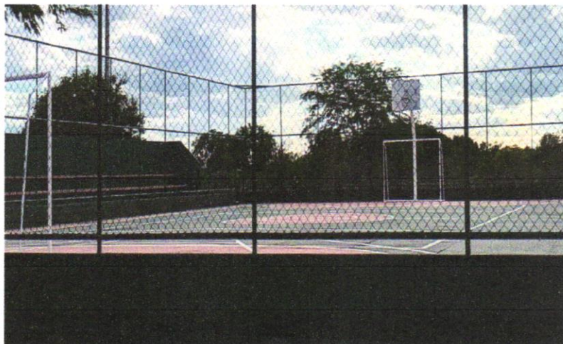
FOTO 03 - Traves oficial para futebol de salão 3x2m em aço galv.3", com requadro e redes de polietileno fio 4mm (conjunto p/futsal)
